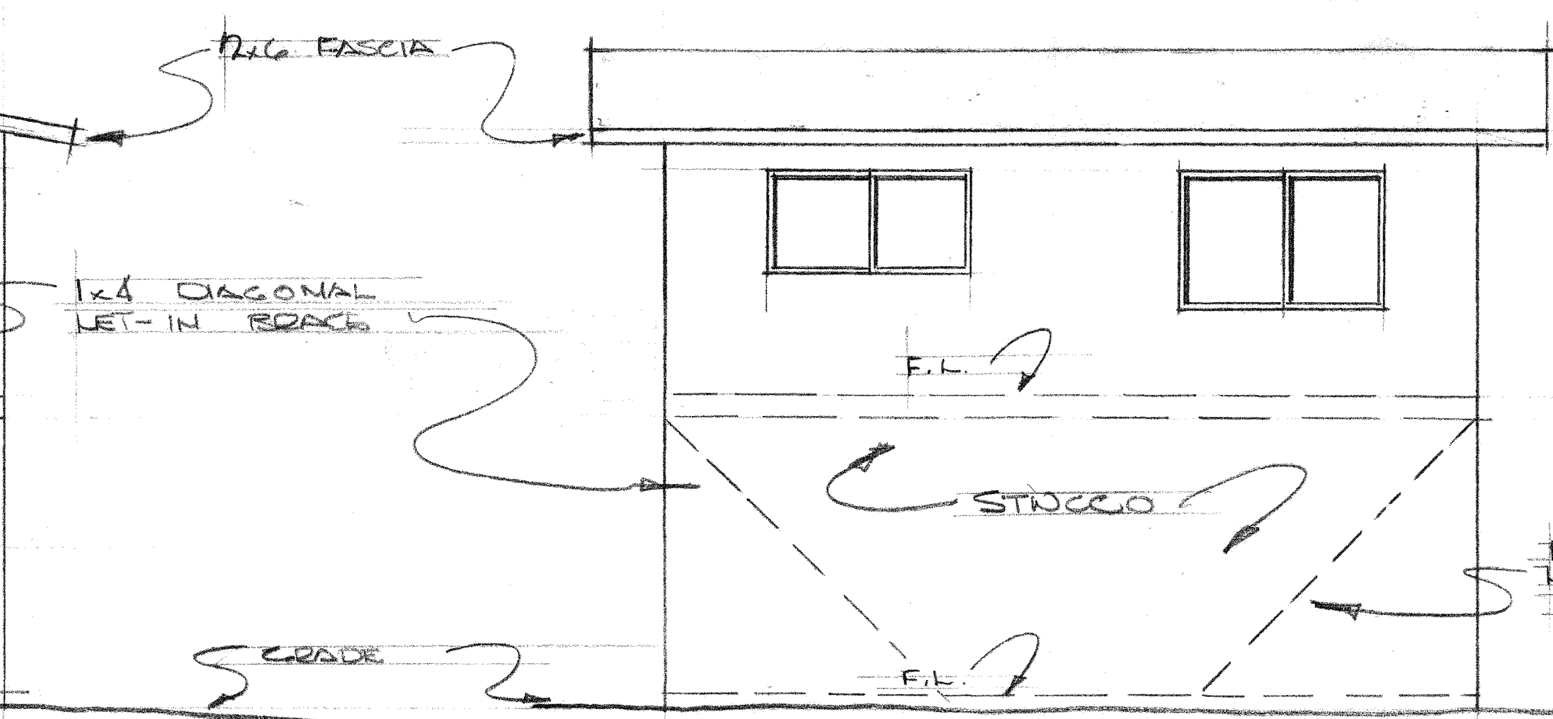
LEFT SIDE
